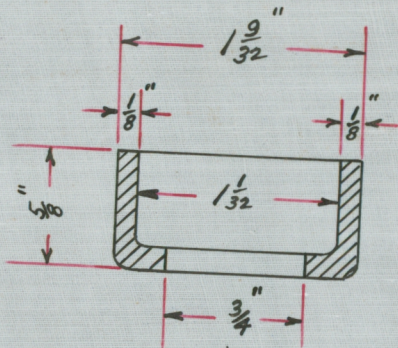
Section thru A-A
